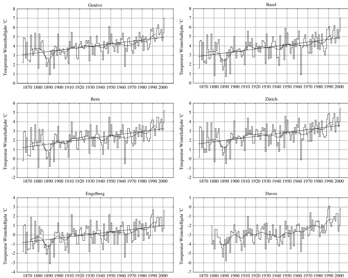
Abbildung 3 (diese und nächste Seite): Langjährige Temperaturentwicklung des Winterhalbjahres. Für jede Station sind die Werte von Jahr zu Jahr, das Mittel über 20 Jahre sowie der lineare Trend (sofern signifikant) angegeben. Die Skalierung umfasst immer 8 Grad Celsius.
