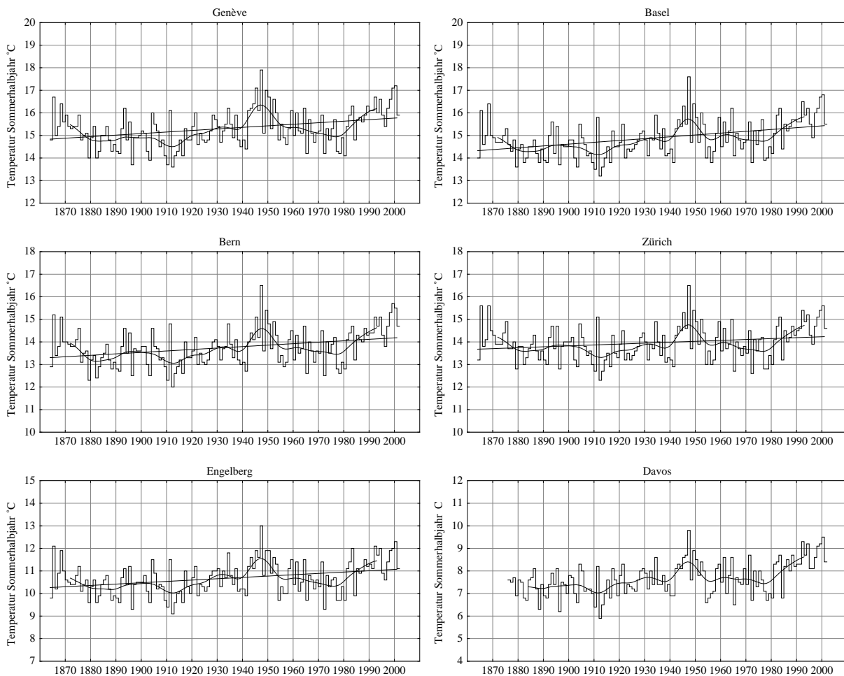
Abbildung 4 (diese und nächste Seite): Langjährige Temperaturentwicklung des Sommerhalbjahres. Für jede Station sind die Werte von Jahr zu Jahr, das Mittel über 20 Jahre sowie der lineare Trend (sofern signifikant) angegeben. Die Skalierung umfasst immer 8 Grad Celsius.
