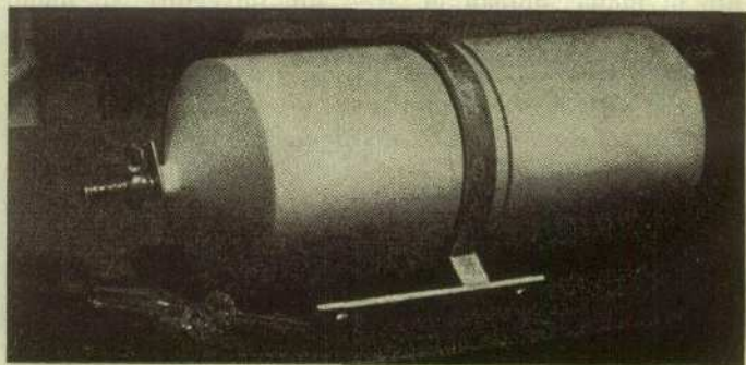
Le pluviototalisateur MZA, dernier modèle: hauteur totale 50 cm; ouverture 200 cm 2 ; contenance équivalant à 400 mm de pluie.
